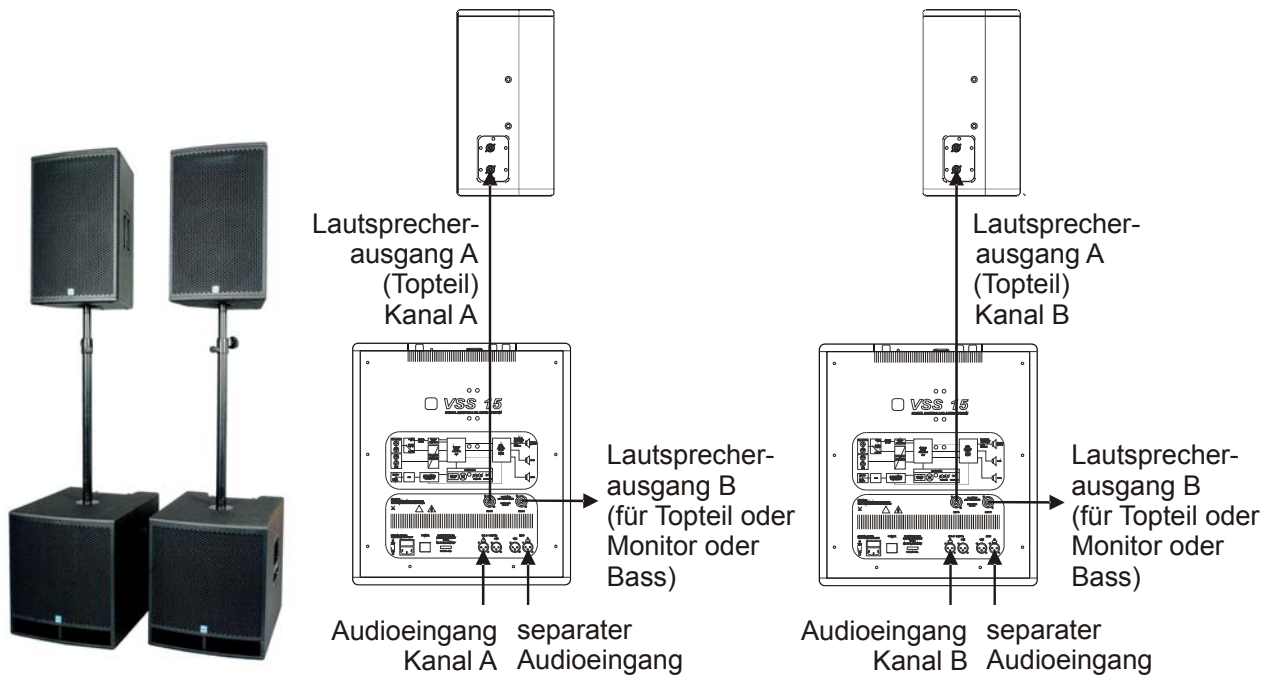
Anschlussschema der SD 4: jeweils vom Lautsprecherausgang „OUT A“ der VSS 15 in das Topteil, die Lautsprecherausgänge „OUT B“ können als Monitorweg bzw. als Delay-Line oder als Basserweiterung belegt werden (vom eingestellten Preset abhängig)
